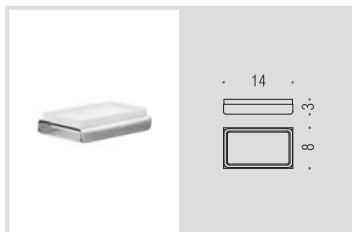
B7040 Porta sapone d'appoggio Standing soap dish holder
